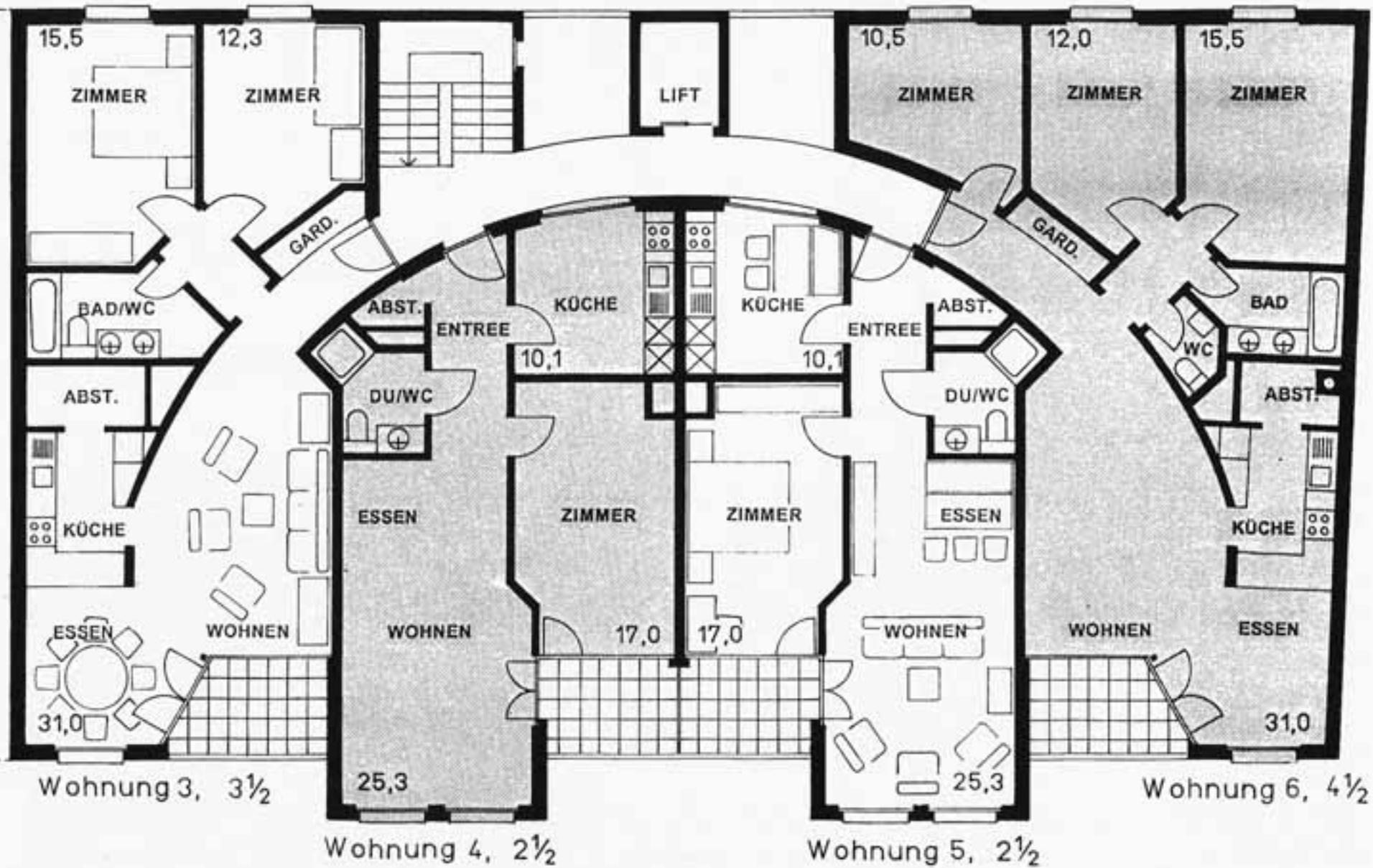
HAUS 38, ERDGESCHOSS.
