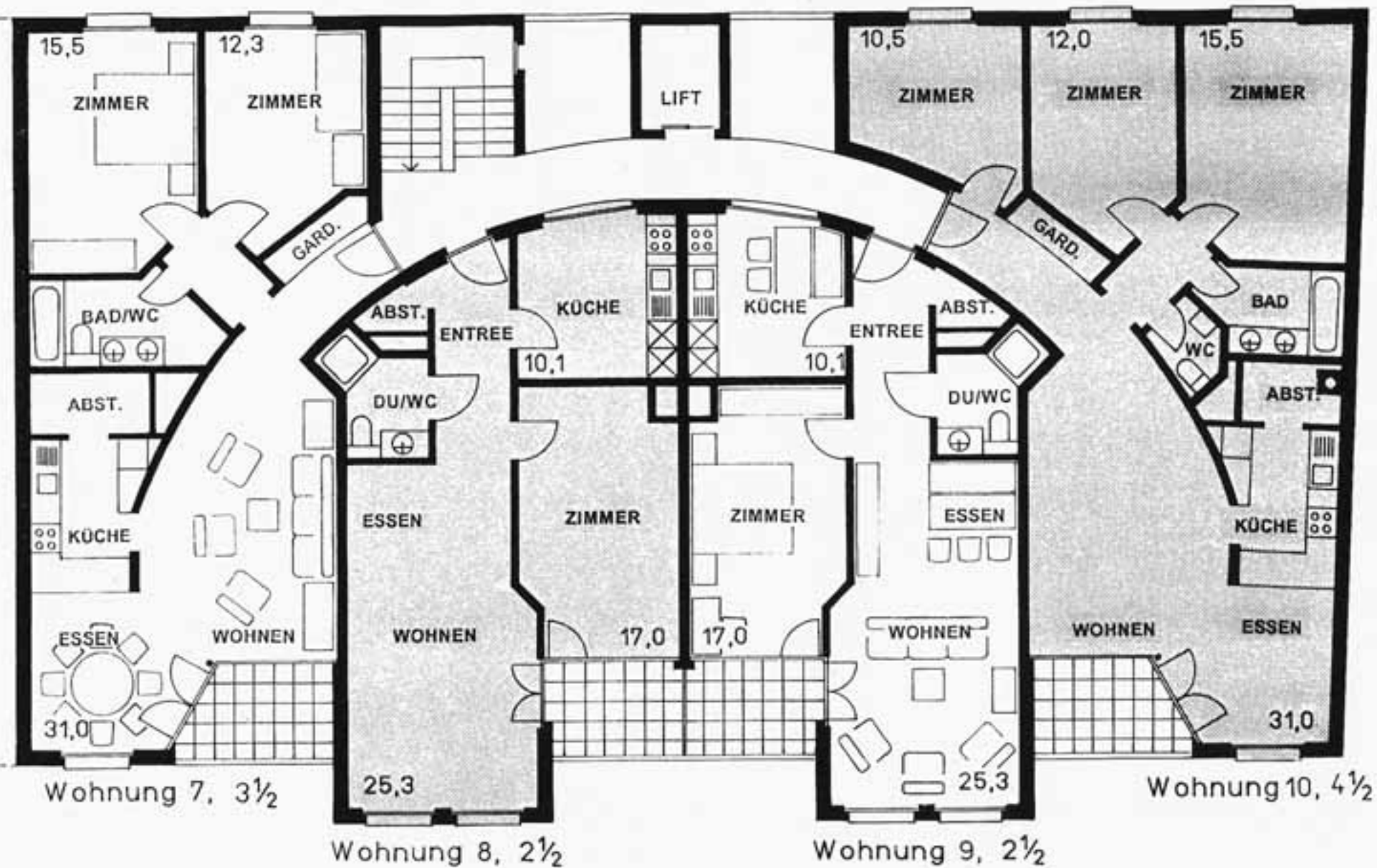
HAUS 38, 1.OBERGESCHOSS.
